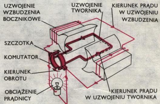
Rys. 9.4. Schemat prądnicy prądu stałego
